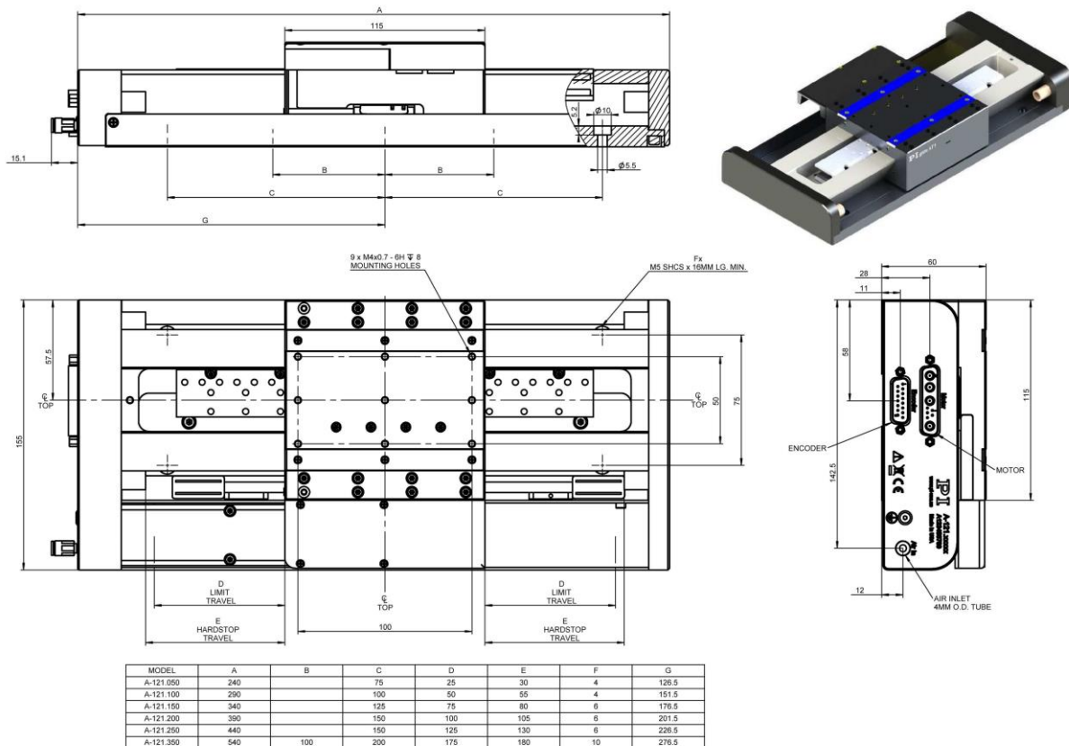
A-121, 尺寸单位为毫米
