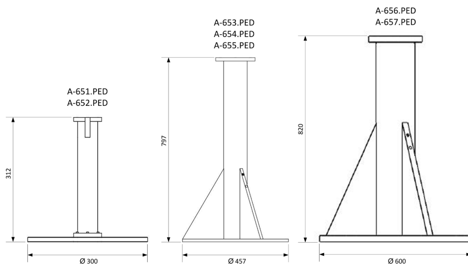
A-65x.PED, 尺寸单位为毫米
